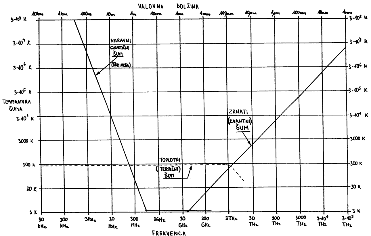
Slika 2.1 – Naravni šumi v radijskih zvezah.
