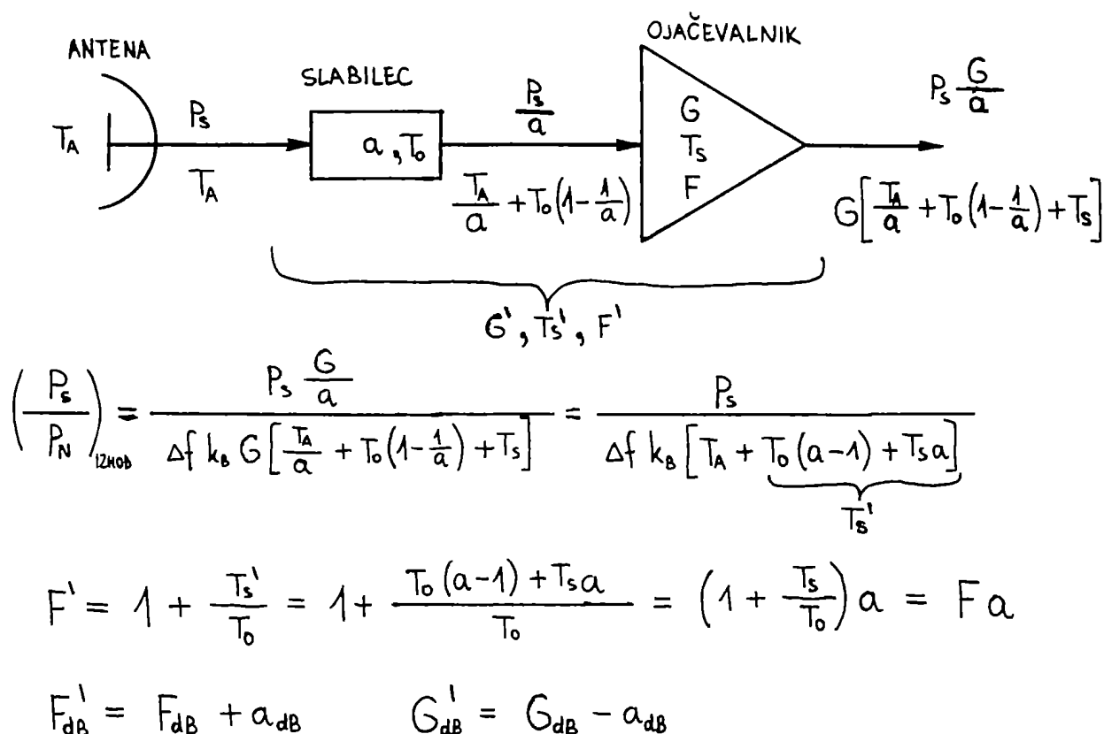
slika 2.11 - vezava slabilca pred ojačevalnikom.
